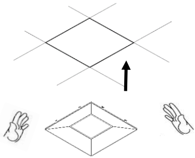
Rys. 1 Sposób zabezpieczenia kołnierza podtynkowego w suficie
