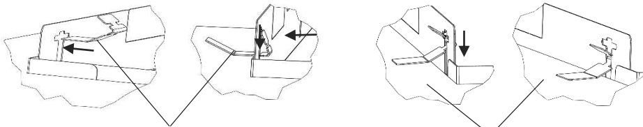
Rys. 1 Sposób zabezpieczenia kołnierza podtynkowego w suficie
