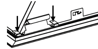
Rys. 2 Sposób zabezpieczenia oprawy bazowej w ramce, przed montażem w kołnierzu podtynkowym NEO.
