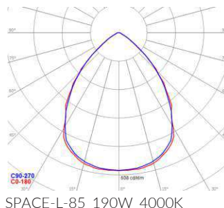
SPACE-L + UCHWYT-G-SPACE-I
