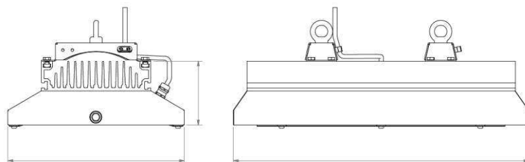
SPACE-L + UCHWYT-G-SPACE-I
