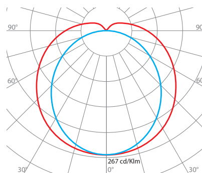
Křivka rozptýlu světla zářivky ECO LT cd/klm — C0 - C180 — C90 - C270
