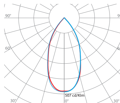
Křivka světelného toku zvoleného osvětlení I-SPOT cd/klm — C0 - C180 — C90 - C270
