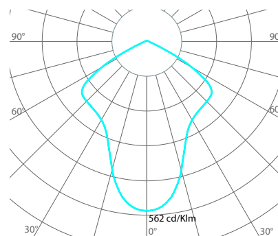
Křivka světelného toku zvoleného osvětlení ROLL cd/klm — C0 - C180/ C90 - C270
