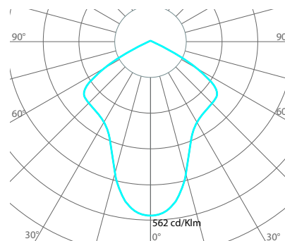
Křivka světelného toku zvoleného osvětlení ROLL-M-X cd/km C0 - C180/ C90 - C270
